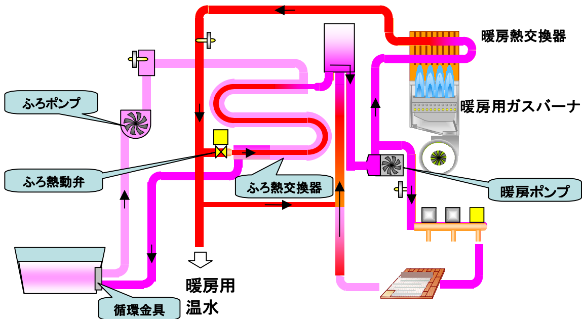
給湯暖房用熱源機の作動原理
